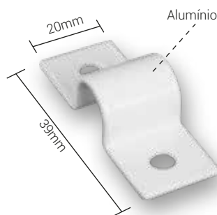
Contra trinco para 1519 e 1521
